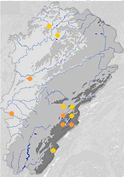
Répartition de la Marouette ponctuée en Franche-Comté en période de nidification (2000-2010)
